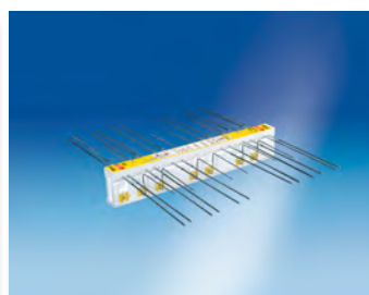
Rupteur pour liaison béton/béton En Isolation Thermique Extérieure et/ou Répartie
